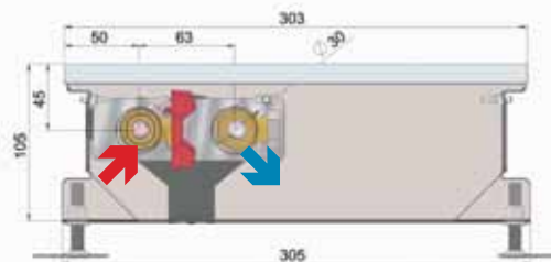
поперечный разрез
