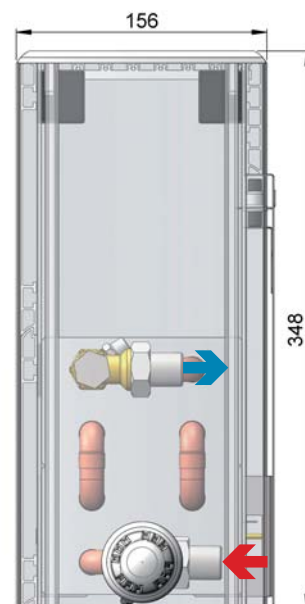
поперечное сечение
